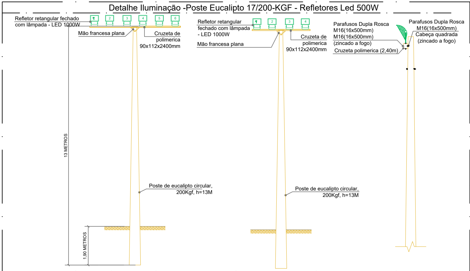
CAMPO DE FUTEBOL POSTES DE ILUMINAÇÃO ESCALA: 1/250
